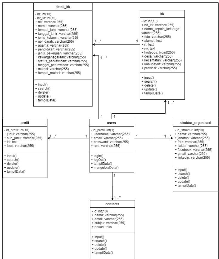
Gambar 4. Class Diagram Data Kependudukan
