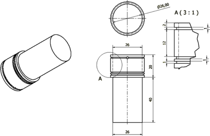
Gambar 7. Piston Panas
