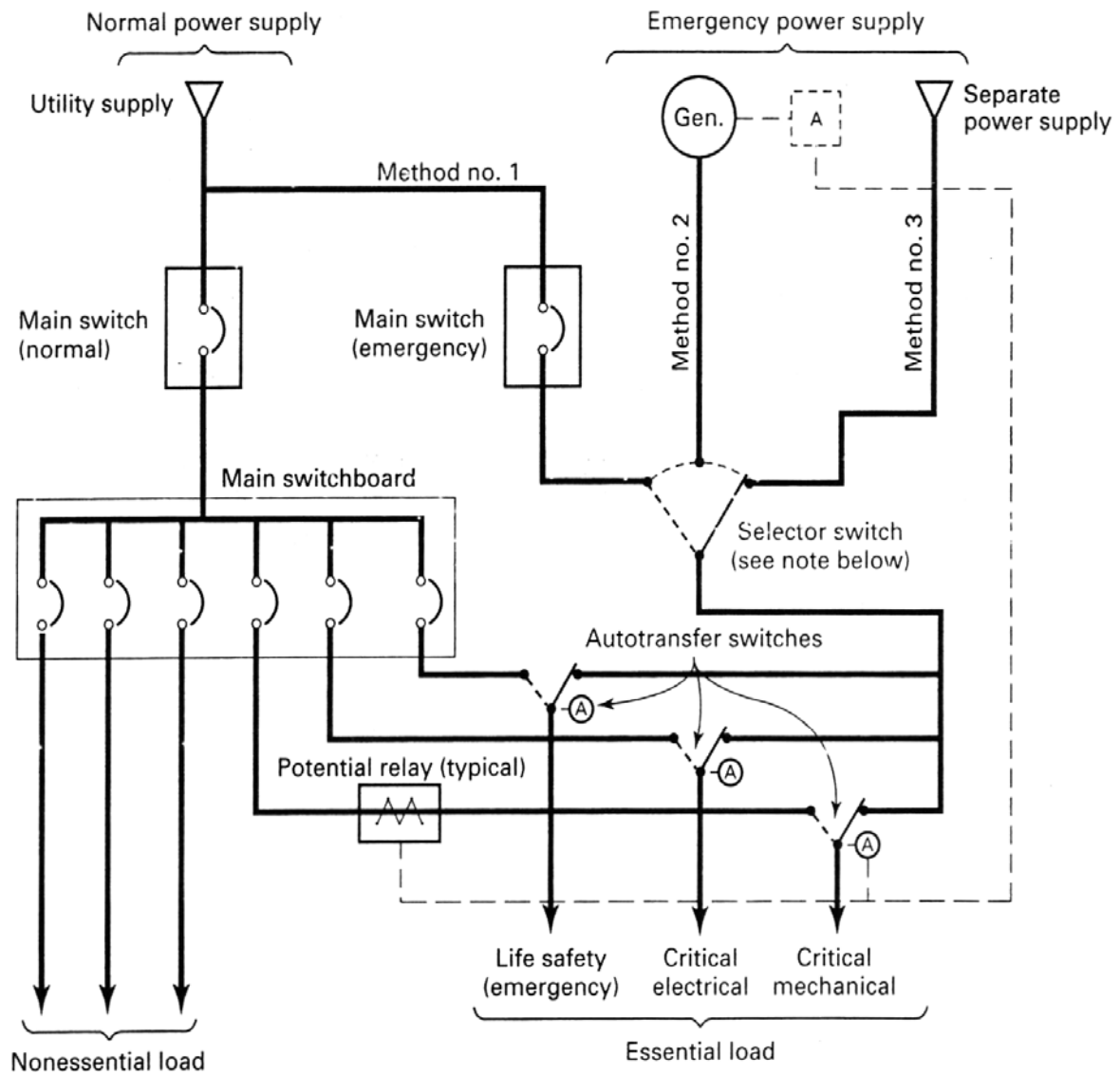
Gambar 1 Sistem Catu Daya Listrik Darurat (Sumber Tao & Janis, 1997)
