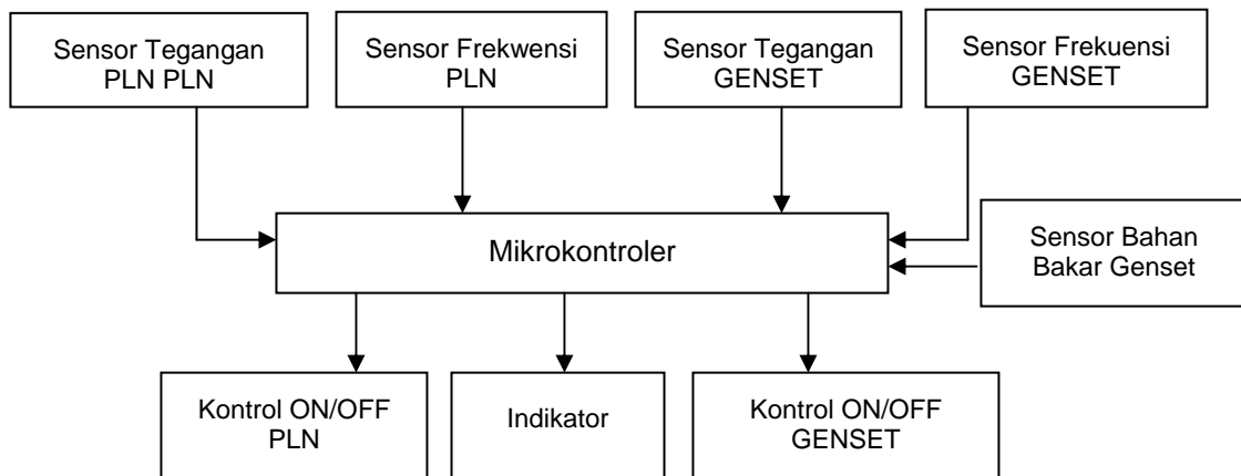
Gambar 4 Diagram Blok Sistem AMF Berbasis Mikrokontroller
