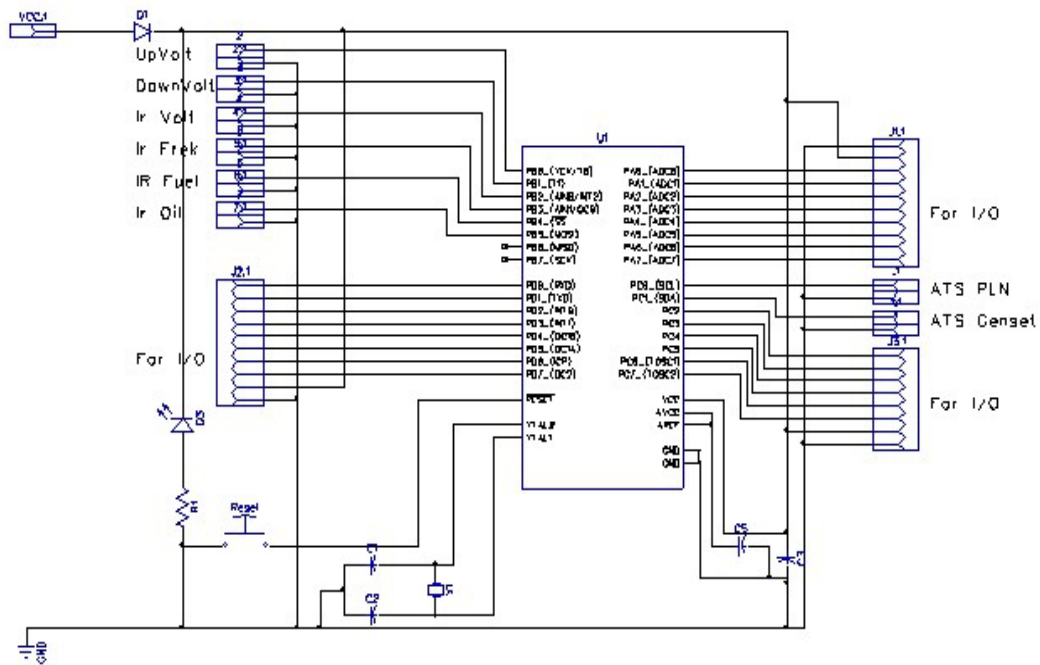
Gambar 5 Rangkaian AMF Berbasis Mikrokontroler
