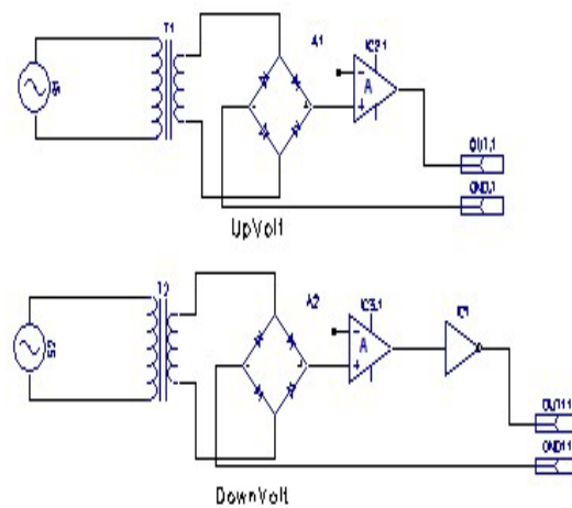
Gambar 6 Rangkaian Sensor Tegangan di PLN dan Genset
