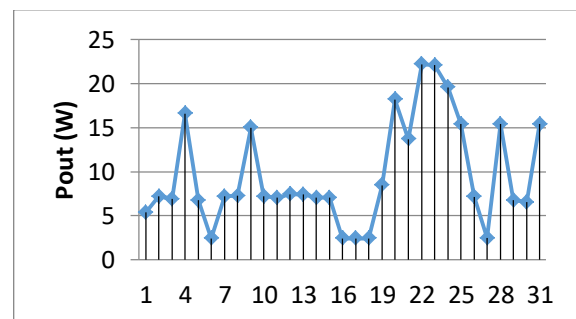
Gambar 10. Grafik hubungan antara daya listrik yang dihasilkan generator terhadap arus serta tegangan dari Generator
