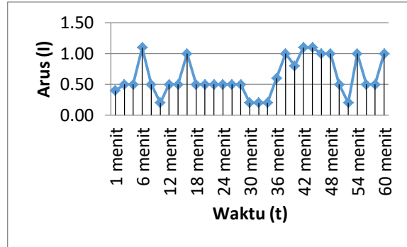
Gambar 8. Grafik Arus (I) dengan Waktu (t) e. Analisis Hasil Pengujian Karakteristik Output Generator
