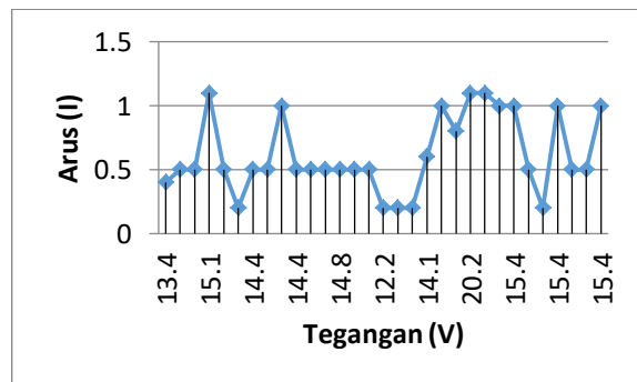
Gambar 9. Grafik hubungan antara arus listrik dengan tegangan listrik yang dihasilkan oleh generator
