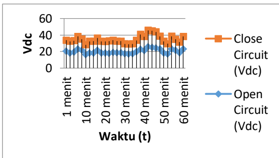
Gambar 7. Grafik Open Circuit (Vdc) dan Close Circuit (Vdc) dengan Waktu (t)
