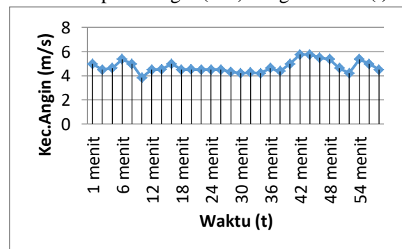
Gambar 6 . Grafik hubungan antara kecepatan angin (m/s) dengan waktu (t)
