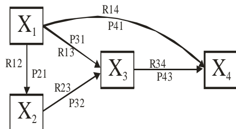
Gambar 1. Desain Penelitian
